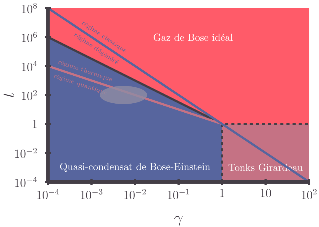
FIGURE 2.4 – Diagramme des régimes principaux du gaz de LL : gaz de Bose idéal, Tonks-Girardeau et qBEC , en fonction des paramètres adimensionnés \gamma et t . Les courbes noires, bleues et orange délimitent les cross-overs entre régimes. La zone grise correspond aux paramètres expérimentaux explorés pendant la thèse. Figure adaptée de [ref_experiment].
